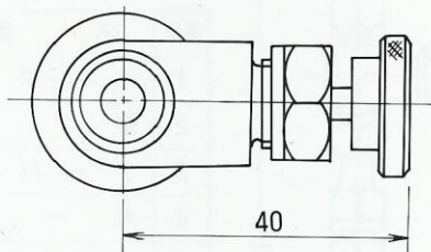
MKDV型
