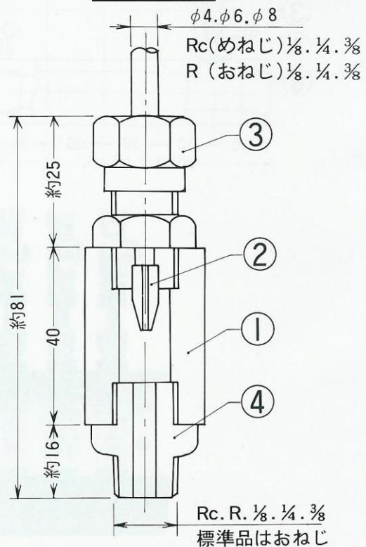
MKD型
